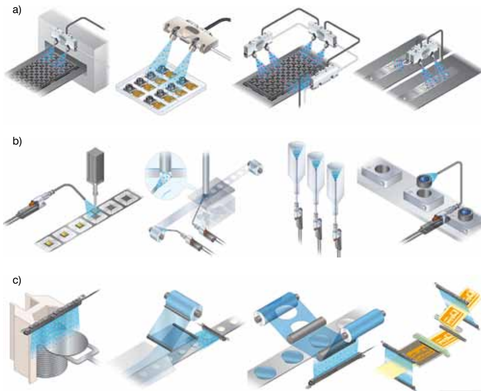
Rys. 3. Możliwości zastosowania jonizatorów: ER-VW (górną), ER-VS (w środku) i ER-X (na dole)
