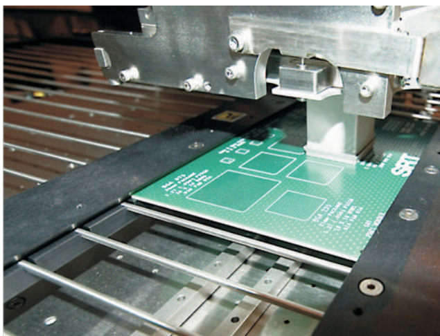
Górny podgrzewacz urządzenia
