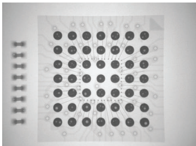
Inspekcja elementu BGA
